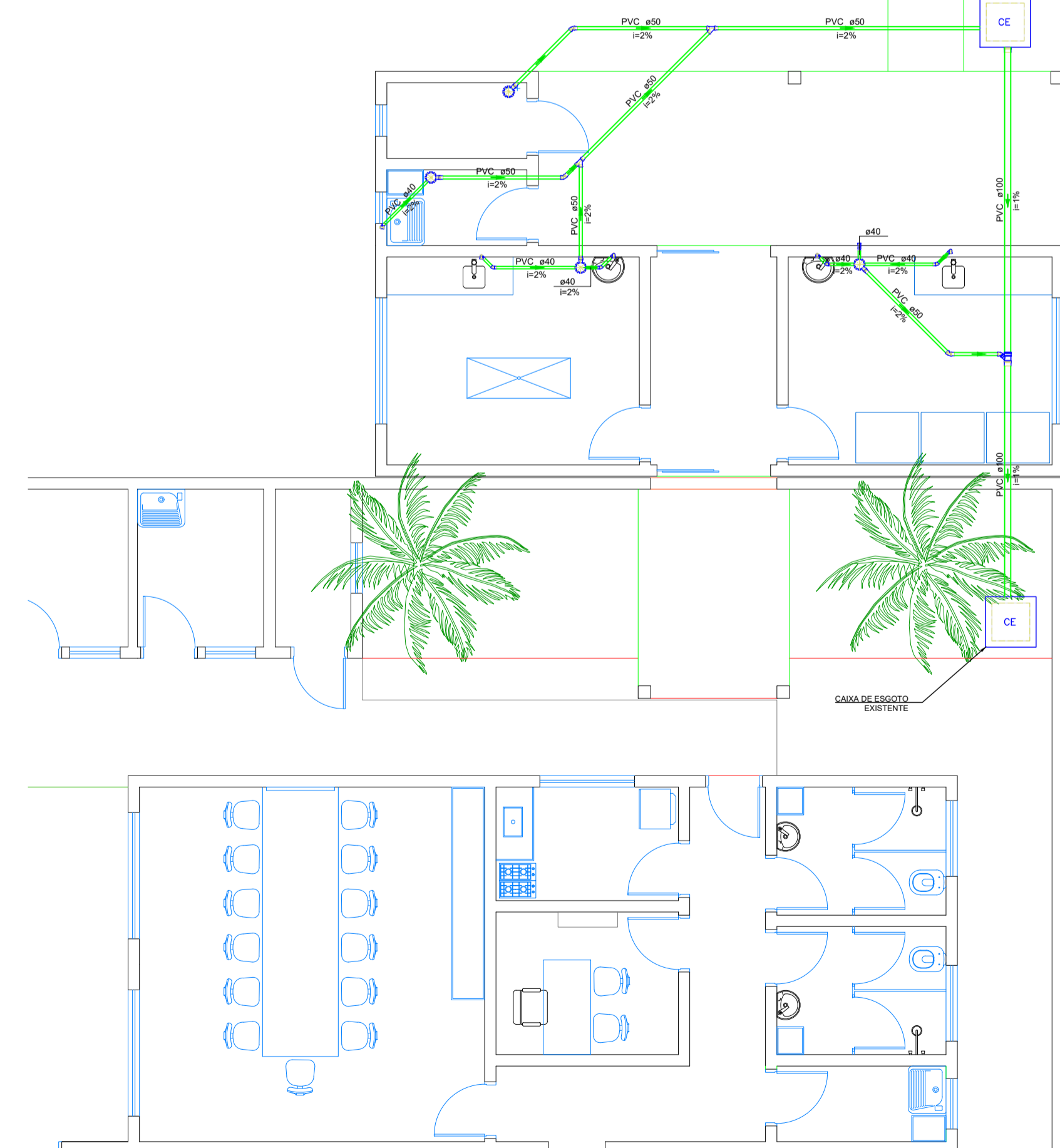
PLANTA BAIXA-ESGOTO ESC: 1/75
