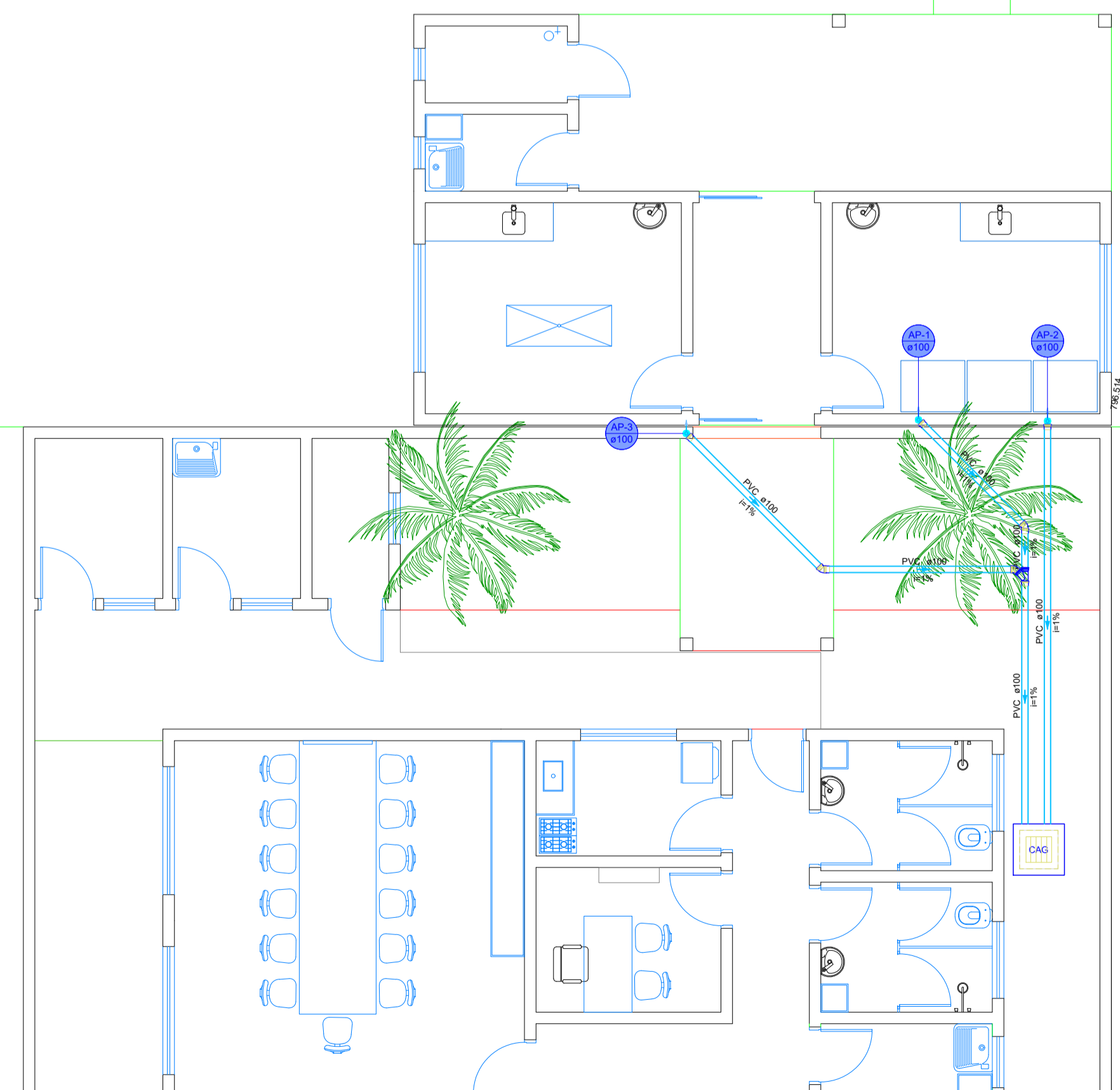
PLANTA BAIXA-ÁGUA FRIA ESC: 1/75
