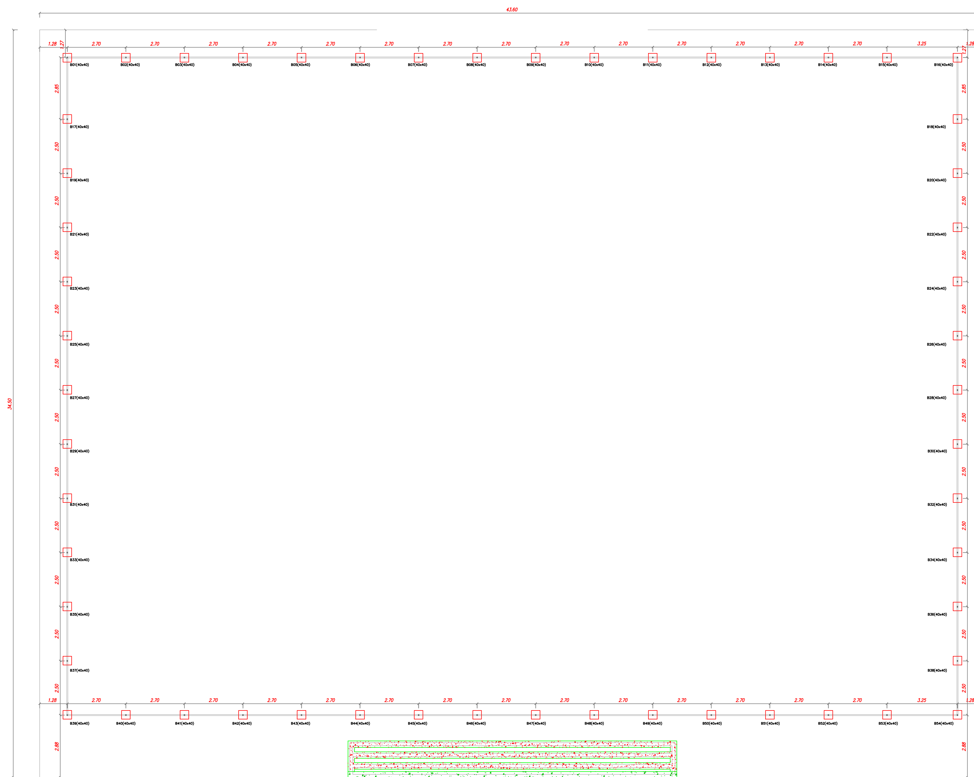
LOCAÇÃO DA FUNDAÇÃO CORRIDA ESCALA _____ 1/100
