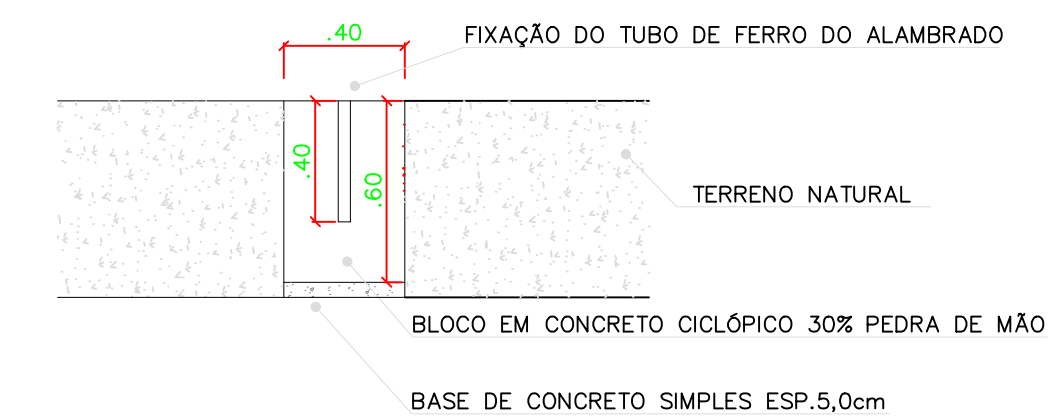
CORTE DO BLOCO DO ALAMBRADO ESC. 1/25
