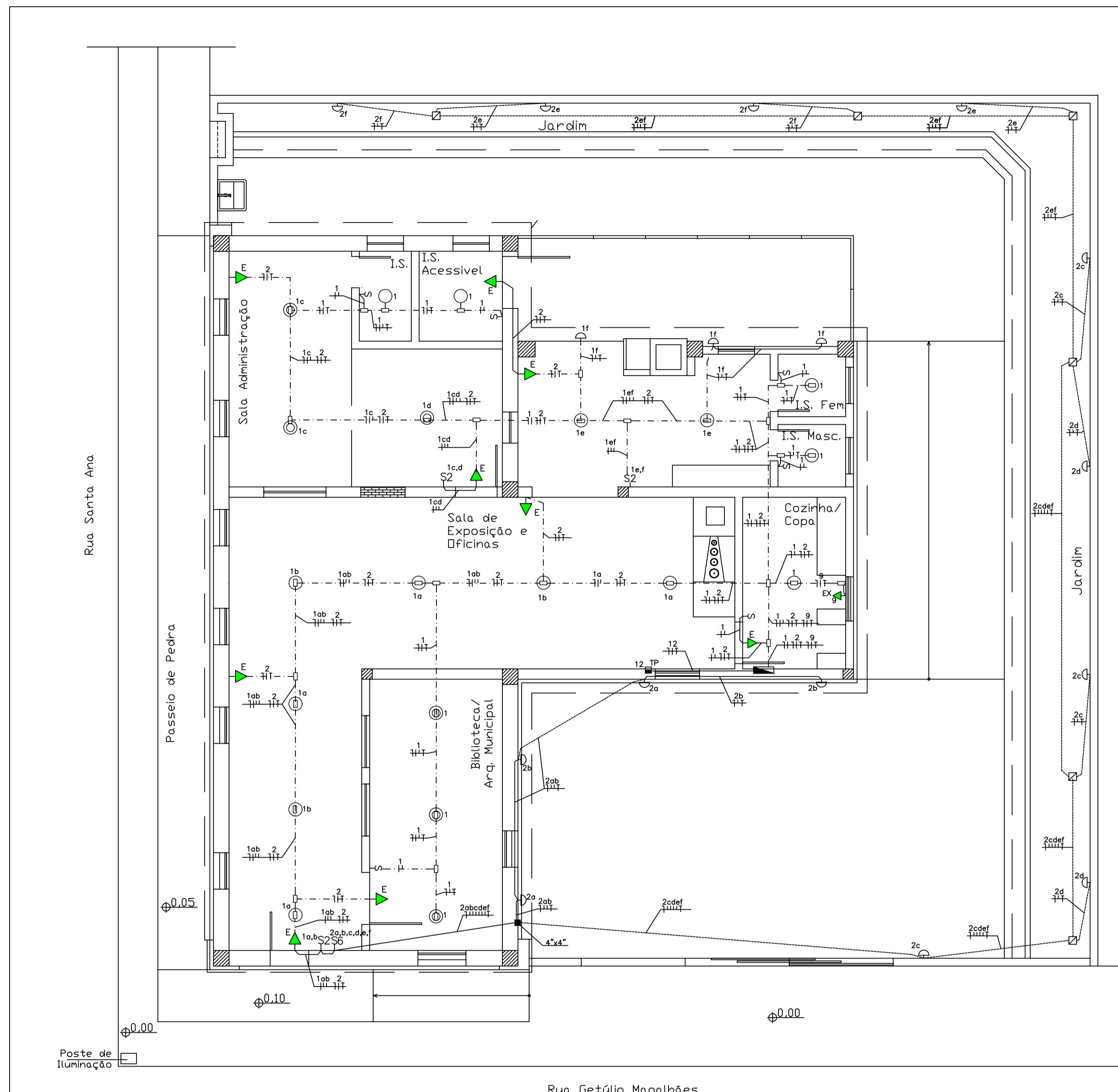
PLANTA - ILUMINAÇÃO ESCALA 1:50
