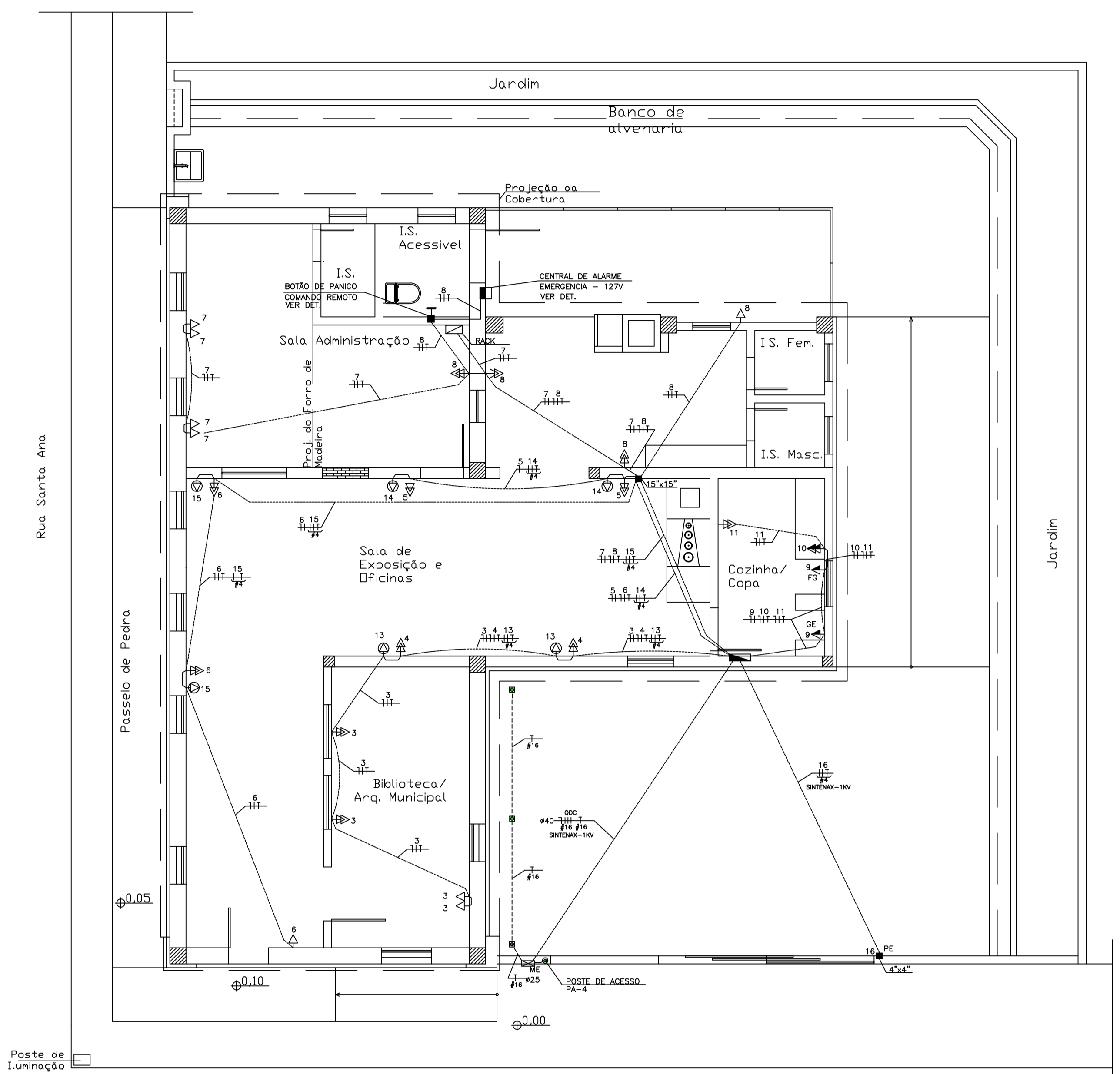
PLANTA - TOMADAS E FORÇA ESCALA 1:50
